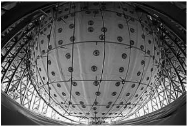
江门中微子实验中心探测器。新华社发
