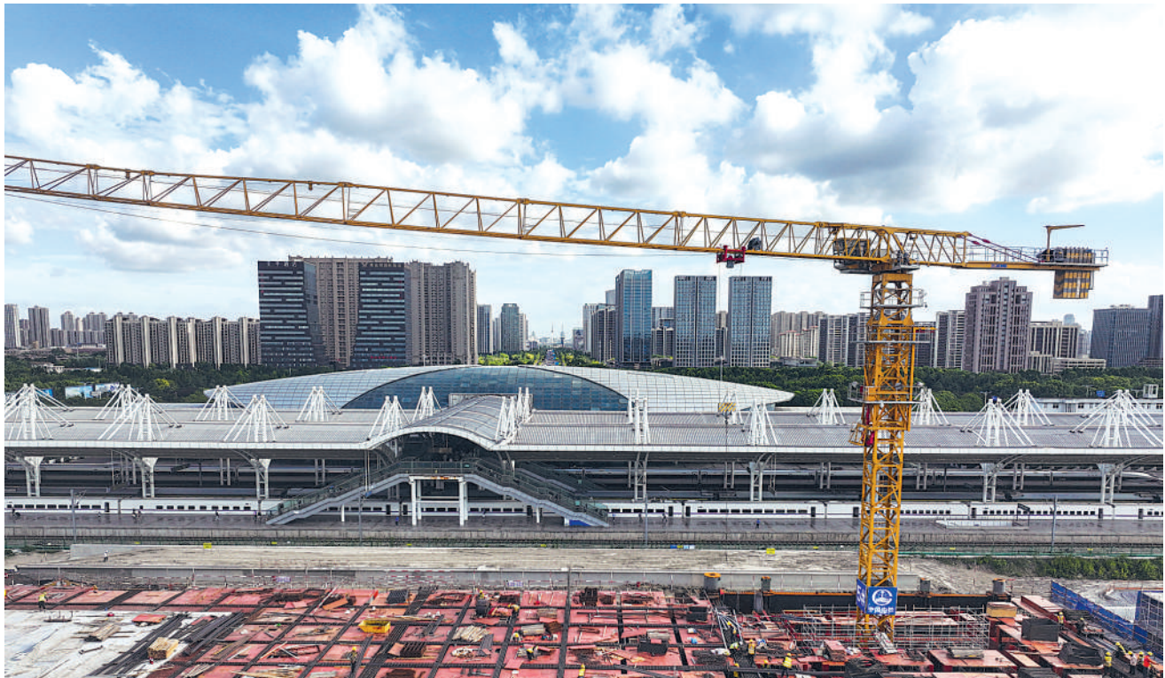
目前，由中铁建工承建的新建上海至南京至合肥高速铁路南通站站房施工有序推进，高架站房B区主体结构完成，侧式站房地板建设完成过半。图为近日拍摄的南通站站房施工现场。
