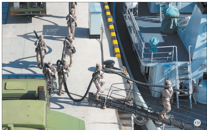
图①:拂晓,油料兵闻令而动。 图②:加油车驶向码头。 图③:为受油舰艇铺设输油管路。 图④:官兵巡查管线设施。 图⑤:进入坑道检查管线。
