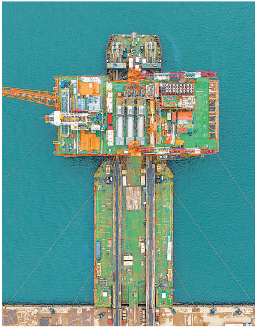
10月13日，中国海上首个多层稠油热采项目——锦州23-2油田开发项目的第二座海上热采平台装船。
